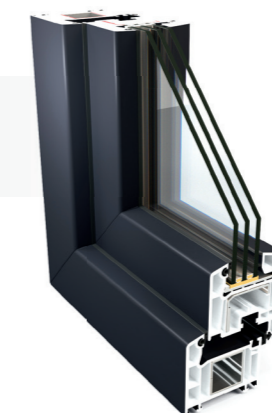
AMBERCLASSIC 70 5/5 KAMMARS
