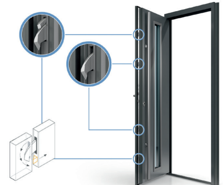
Zasuwnica AV3 z zapadką dzienną
